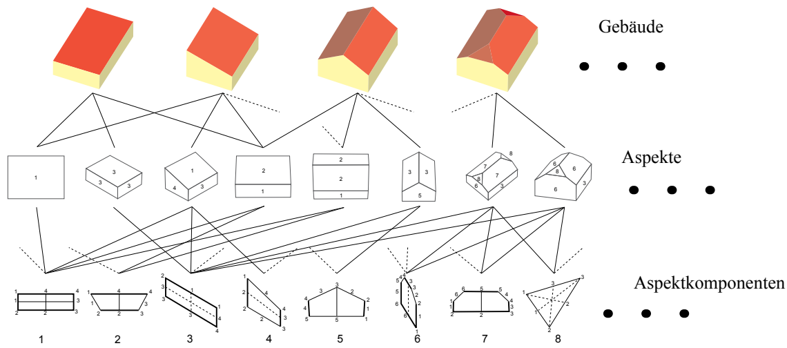
Abbildung 7: Die gebäudespezifische Aspekthierarchie.
