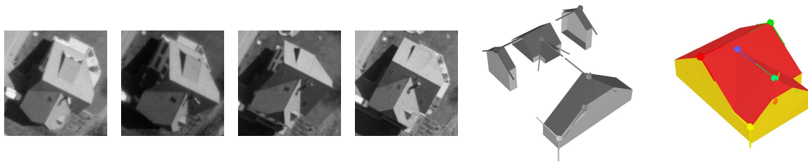
Abbildung 9: Aus vierfach überdeckter Gebäudeabbildung abgeleitete Gebäudekomponenten und daraus generierte Gebäudehypothese.
