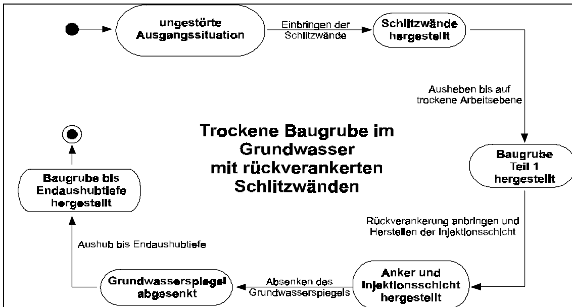
Abb. 4 Dynamisches Modell nach Rumbaugh für die Erstellung einer trockenen Baugrube
