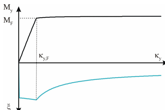
Abb. 7: M- \kappa - \xi Beziehung
