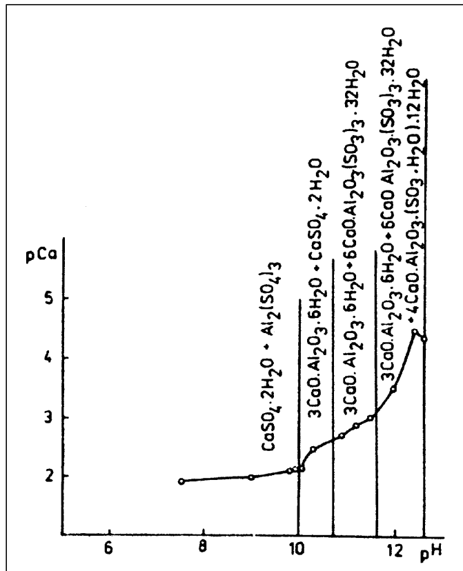
Abb. 16: Abhängigkeit des \text{pCa} ( = -\log c_{\text{Ca}^{2+}} ) vom \text{pH} ( = -\log c_{\text{H}^+} ) mit Informationen über die auftretenden festen Phasen nach [142]
