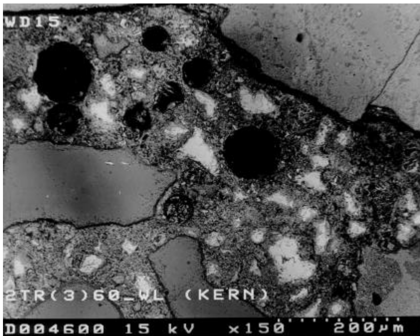
Abb. 78: Gefügebild mit überwiegend von Phasenneubildung freien Poren, Anschliff; REM-Aufnahme von Straßenbeton 2 nach 2. Trocknung der 3. Belastungsstufe
