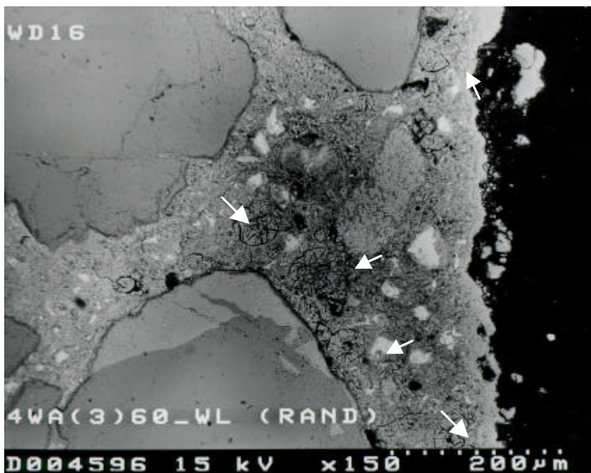
Abb. 79: Gefügebild mit durch Phasenneubildungen verschlossenen Poren, Anschliff; REM-Aufnahme von Straßenbeton 2 nach 4 Wechselzyklen der 3. Belastungsstufe
