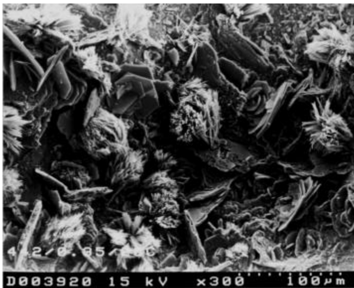
Abb. 42: Ettringitformationen und Monosulfatrossetten in einem Hohlraum; REM-Aufnahme von Feinkornbeton nach 3 Wechselzyklen I. Belastungsstufe ; \text{SO}_3 -Gehalt des Zementes 2,3 %; w/z-Wert 0,35
