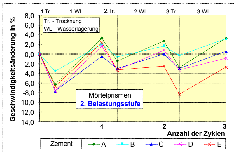
Abb. 104: Ultraschall-Geschwindigkeitsänderung während der Wechsellagerung der 2. Belastungsstufe; Mörtelprismen mit unterschiedlichen Alkaligehalten
