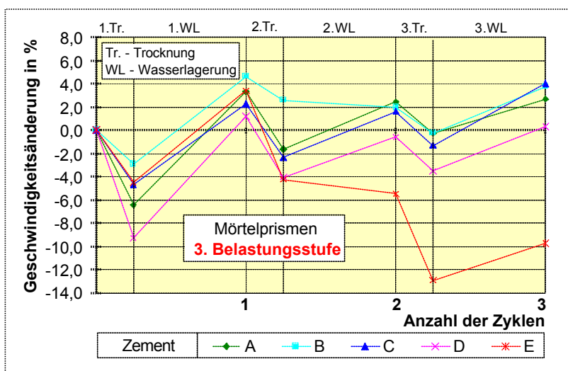
Abb. 105: Ultraschall-Geschwindigkeitsänderung während der Wechsellagerung der 3. Belastungsstufe; Mörtelprismen mit unterschiedlichen Alkaligehalten
