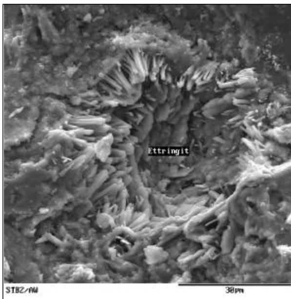
Abb. 85: Ettringitkristalle in einer Luftpore; REM-Aufnahme von Straenbeton 2 nach 2jhriger Nutzung
