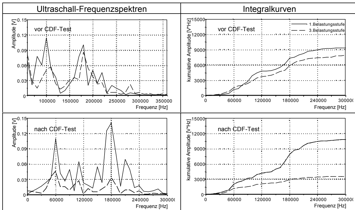
Abb. 92: Ultraschall-Frequenzspektren (links) und Integralkurven (rechts); Straßenbeton 1 nach 4 Wechselzyklen der 1. und 3. Belastungsstufe vor CDF-Test (oben) und nach CDF-Test (unten)
