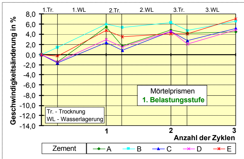
Abb. 103: Ultraschall-Geschwindigkeitsänderung während der Wechsellagerung der 1. Belastungsstufe; Mörtelprismen mit unterschiedlichen Alkaligehalten
