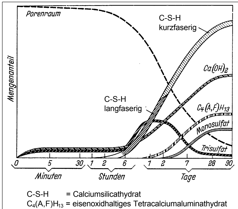
Abb. 14: Schematische Darstellung der Bildung der Hydratphasen und der Gefügeentwicklung bei der Hydratation des Zementes nach [122]
