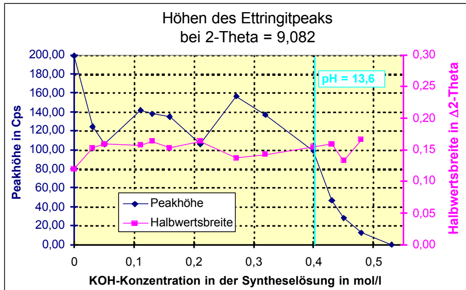
Abb. 138: Auswertung der Röntgenanalysen der Ettringitsyntheseveruche bei unterschiedlichen KOH-Konzentrationen in der Syntheselösung; Höhen und Halbwertsbreiten des Ettringitpeaks bei 2-Theta = 9,082
