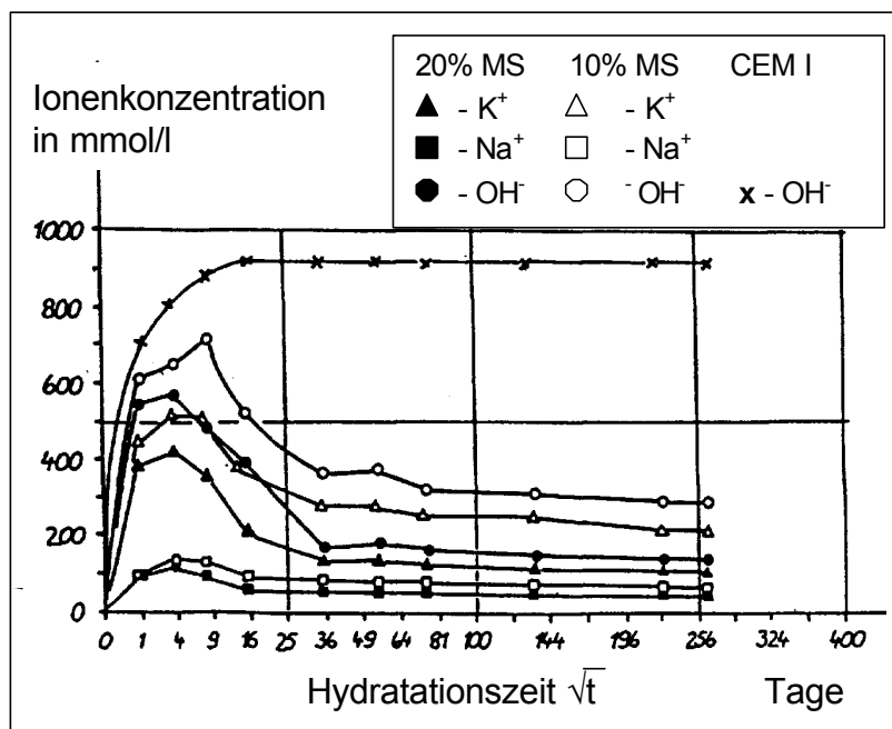
Abb. 19: Chemische Zusammensetzung der Porenlösung von Portlandzement mit 0 % , 10 % und 20 % Microsilica (MS) als Funktion der Hydratationszeit bei 20 °C, w/z = 0,5 [280]
