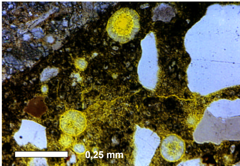
Abb. 50: Ettringitegefüllte Luftporen, die scheinbar einen unterschiedlichen Porenfüllungsgrad aufweisen; Mikroskopische Dünnschliffaufnahme eines nach mehrjähriger Nutzung durch Ribbildung stark geschädigten Straßenbetons
