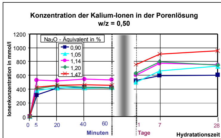
Abb. 121: Veränderung der Kalium -Ionen-Konzentration in der Porenlösung während der Hydratation bei w/z = 0,5 , Zemente A - E mit unterschiedlichen \text{Na}_2\text{O} -Äquivalenten
