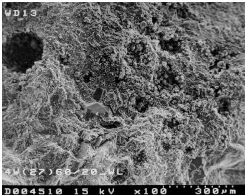
Abb. 73: Ettringitbeläge an der Wandung großer Kugelporen, kleinere Poren sind aufgrund der Porenfüllung nicht mehr identifizierbar; REM-Aufnahme von Straßenbeton 2 nach 4 Wechselzyklen der 2. Belastungsstufe
