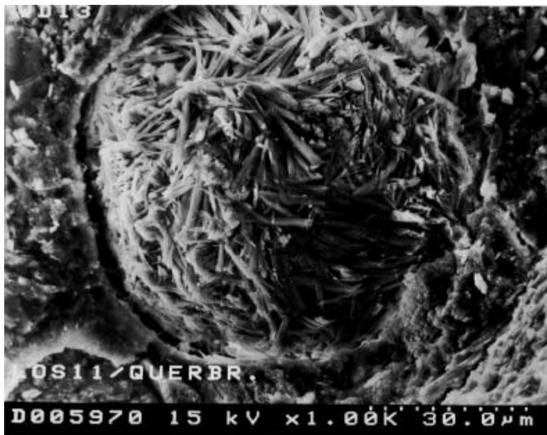
Abb. 51: Vollständig mit Ettringitkristallen gefüllte Luftpore; REM-Aufnahme der Bruchfläche eines nach mehrjähriger Nutzung durch Ribbildung stark geschädigten Straßenbetons
