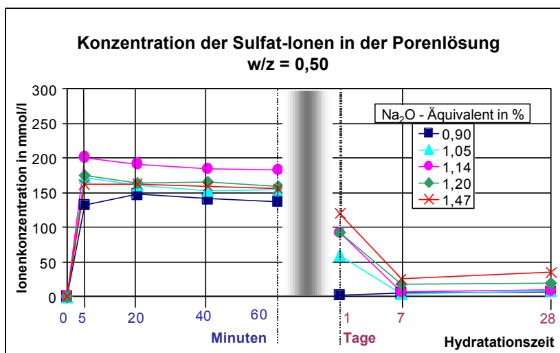
Abb. 125: Veränderung der Sulfat-Ionen-Konzentration in der Porenlösung während der Hydratation bei w/z = 0,5 ; Zemente A - E mit unterschiedlichen \text{Na}_2\text{O} -Äquivalenten (A: 0,9 %; B: 1,05 %; C: 1,14 %; D: 1,20 %; E: 1,47 %)
