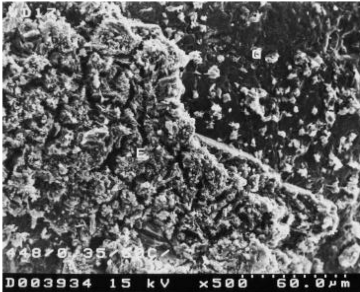
Abb. 45: Ettringitschicht auf der Oberfläche eines Quarzkorns REM-Aufnahme von Feinkornbeton nach 3 Wechselzyklen III. Belastungsstufe; SO 3 -Gehalt des Zementes 2,3 %; w/z-Wert 0,35
