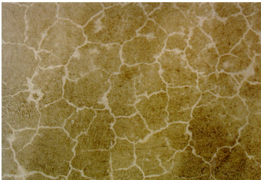
Abb. 1: Makroskopisches Schadensbild einer Betonoberfläche - map cracking (grobkristalliner Ettringit in Schwachstellen des Gefüges nachweisbar)
