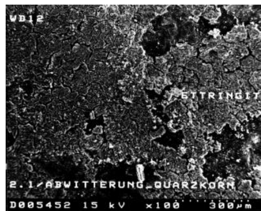
Abb. 91: REM-Aufnahme
