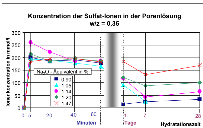
Abb. 126: Veränderung der Sulfat-Ionen-Konzentration in der Porenlösung während der Hydratation bei w/z = 0,35 ; Zemente A - E mit unterschiedlichen \text{Na}_2\text{O} -Äquivalenten (A: 0,9 %; B: 1,05 %; C: 1,14 %; D: 1,20 %; E: 1,47 %)
