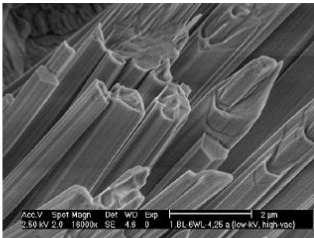
Abb. 152: Nadelförmige Ettringitformationen, die aus Schichten dicht aneinanderliegender feiner Ettringitkristalle aufgebaut sind; ESEM-Aufnahme eines Straßenbetons ( ohne Kohlenstoff-Bedampfung)
