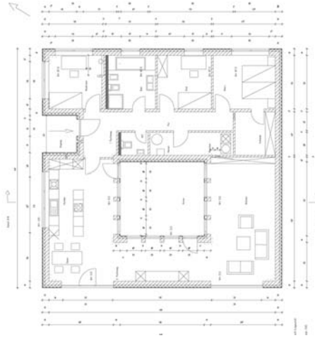
Abb. 225 Grundriss
