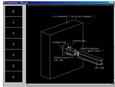
Abb. 83 Konstruktionsdetail
