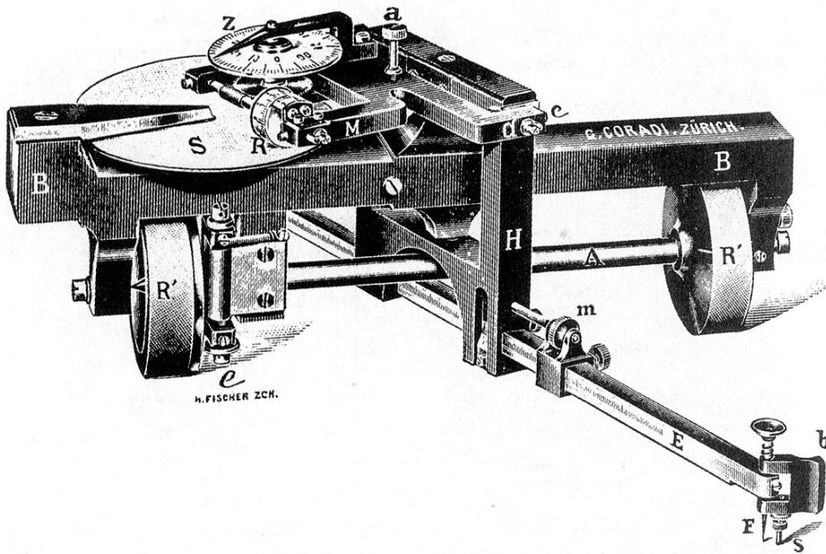
Planimeter
