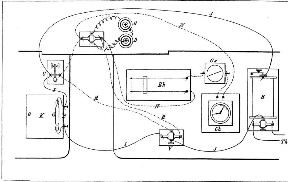
Schaltplan zur Reaktionszeitmessung von Max Friedrich
