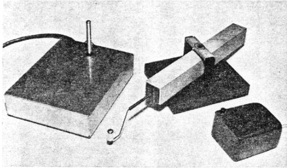
Engelbarts Devices: Grafacon, Maus, Lightpen und Knee Control (an Sekretärinnenbein) unten: Zielerfassung beim Autofahren (Studie von Daimler Benz, Herbst 1998)
