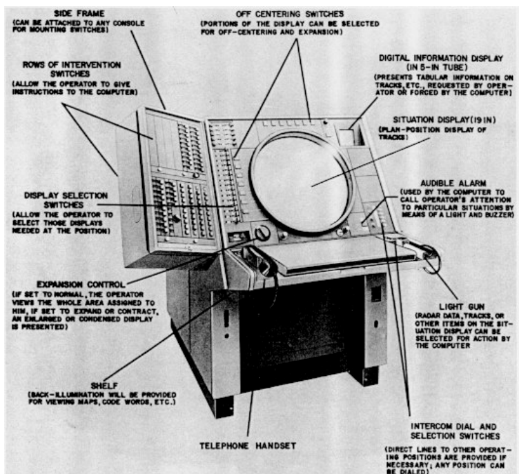
SAGE Kontrollzentrum und SAGE-Konsole
