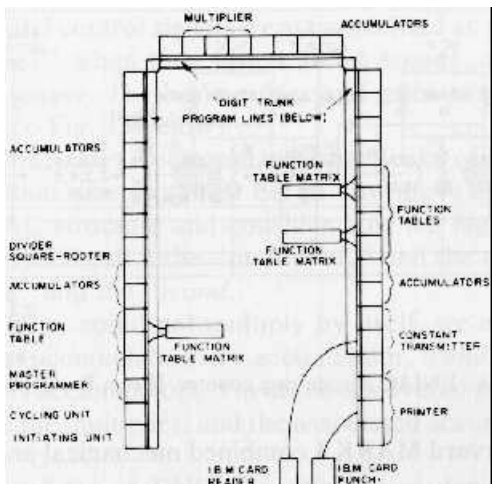
Ausschnitte aus dem Lageplan der Einheiten des ENIAC
