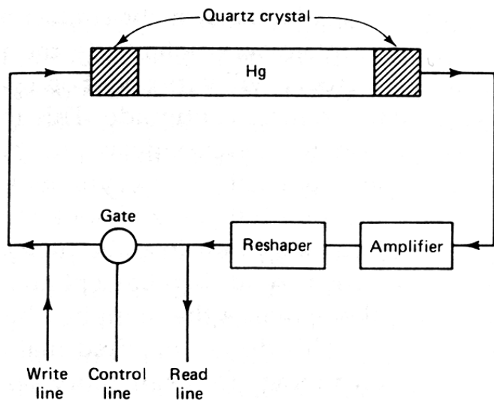
Prinzipschaltung einer Delay Line, auf Vorschlag Turings auch mit Gin zu betreiben
