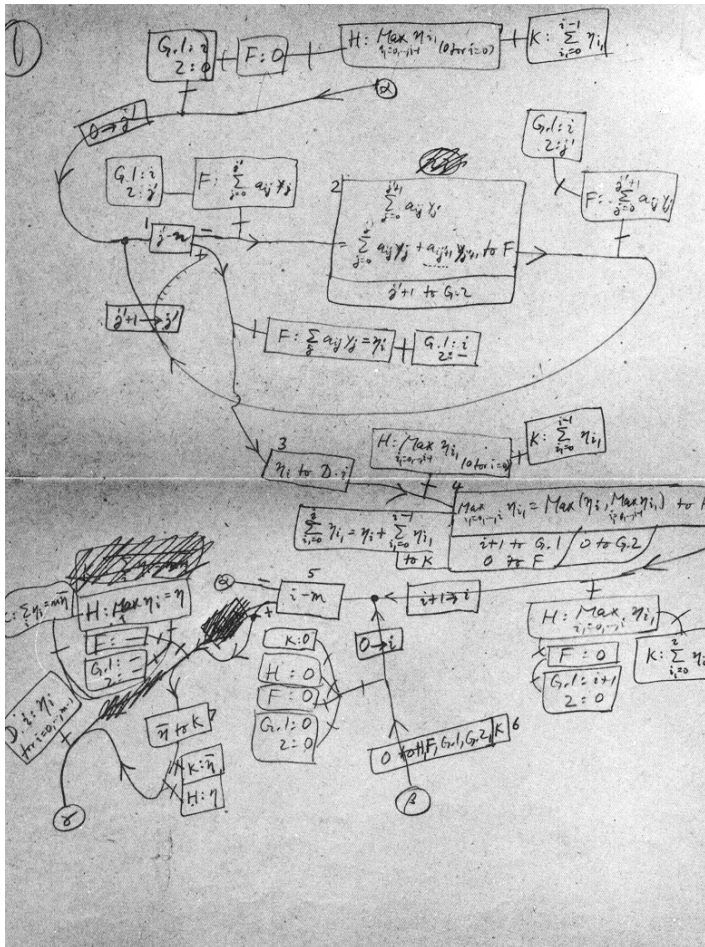
Flowchart-Skizze John von Neumanns für den LAS- Rechner zu einem von E. W. Paxson formulierten Problem (Duell zwischen einem Zerstörer und einem U-Boot)
