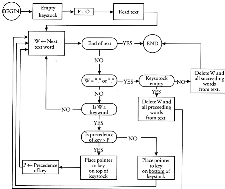
»ELIZA« Flußdiagramm
