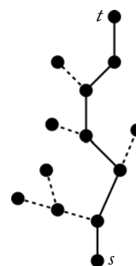
Fig. 8: Ein Baum
