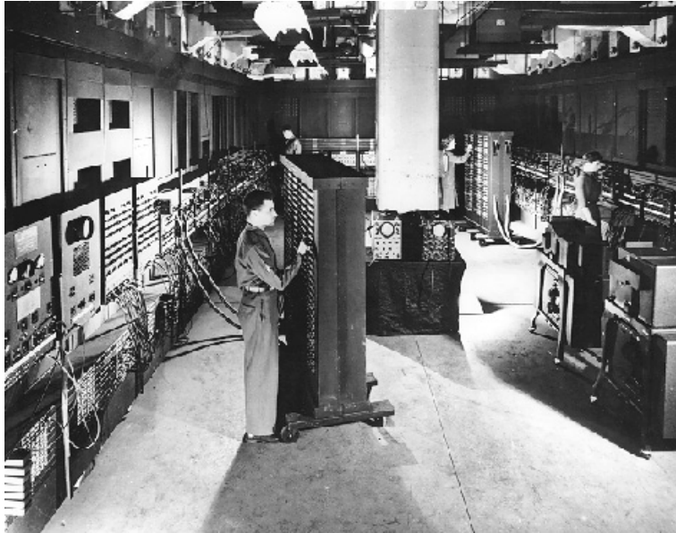
Die U-förmige Anlage des ENIAC und girls beim Verdrabten der Einheiten («proper programming»)
