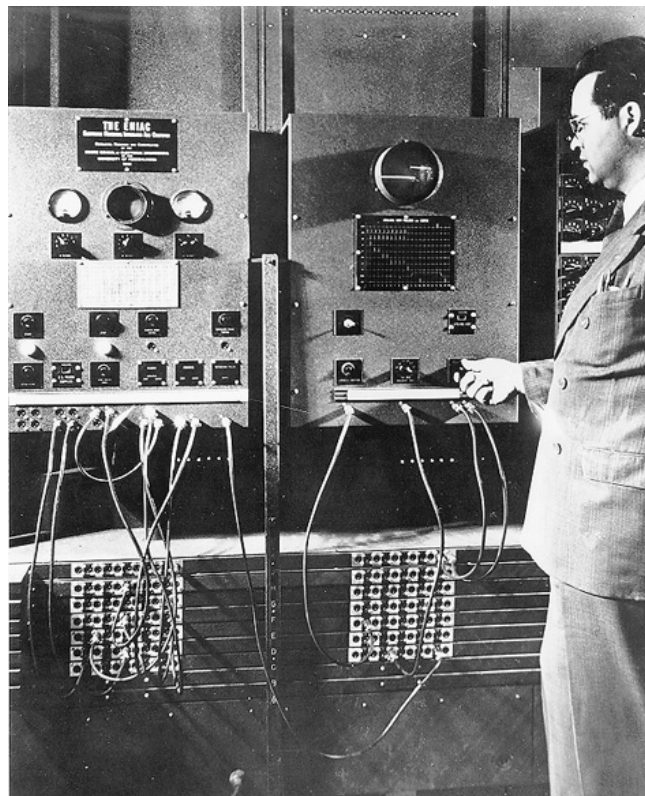
Die Cycle-Unit des ENIAC (100kHz)
