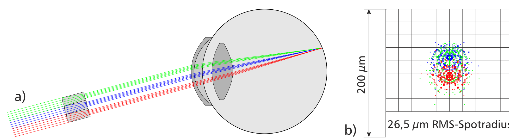
Abb. 4: Kanalübergreifendes Optikdesign mit ZEMAX™. a) Systemlayout mit drei Segmenten. b) Gesamtspot der drei Kanäle.
