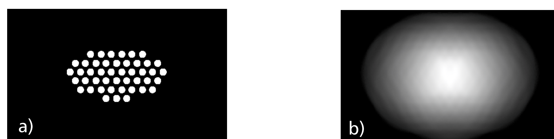
Abb. 3: Gesamtheit als Summe der einzelnen Kanäle. a) Blendenarray. b) Resultierende Helligkeitsverteilung.
