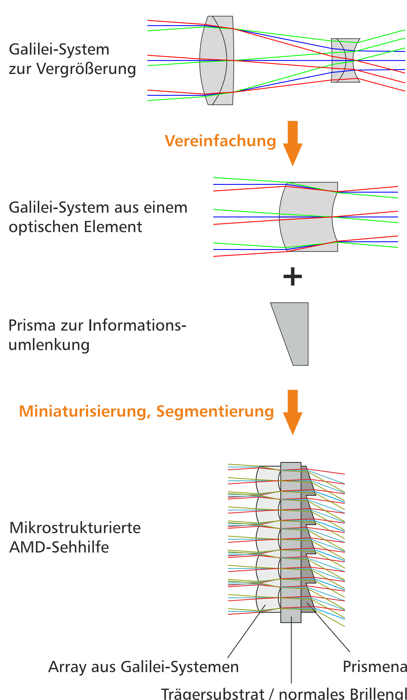
Abb. 2: Realisierungsprinzip auf Basis von Arrayoptiken
