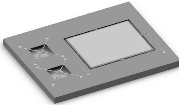
Abbildung 1: Schematische Darstellung des Sensors, links die beiden Gassensoren und rechts der Feuchtesensor auf jeweils separaten Hotplates.
