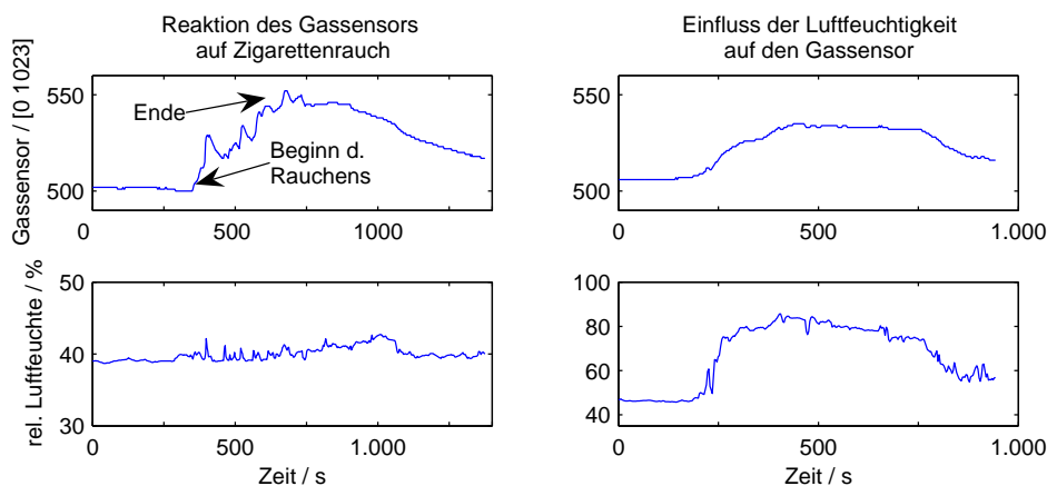
Abbildung 2: Links: Reaktion des Gassensors auf Zigarettenrauch, rechts Reaktion auf Luftfeuchtigkeit.
